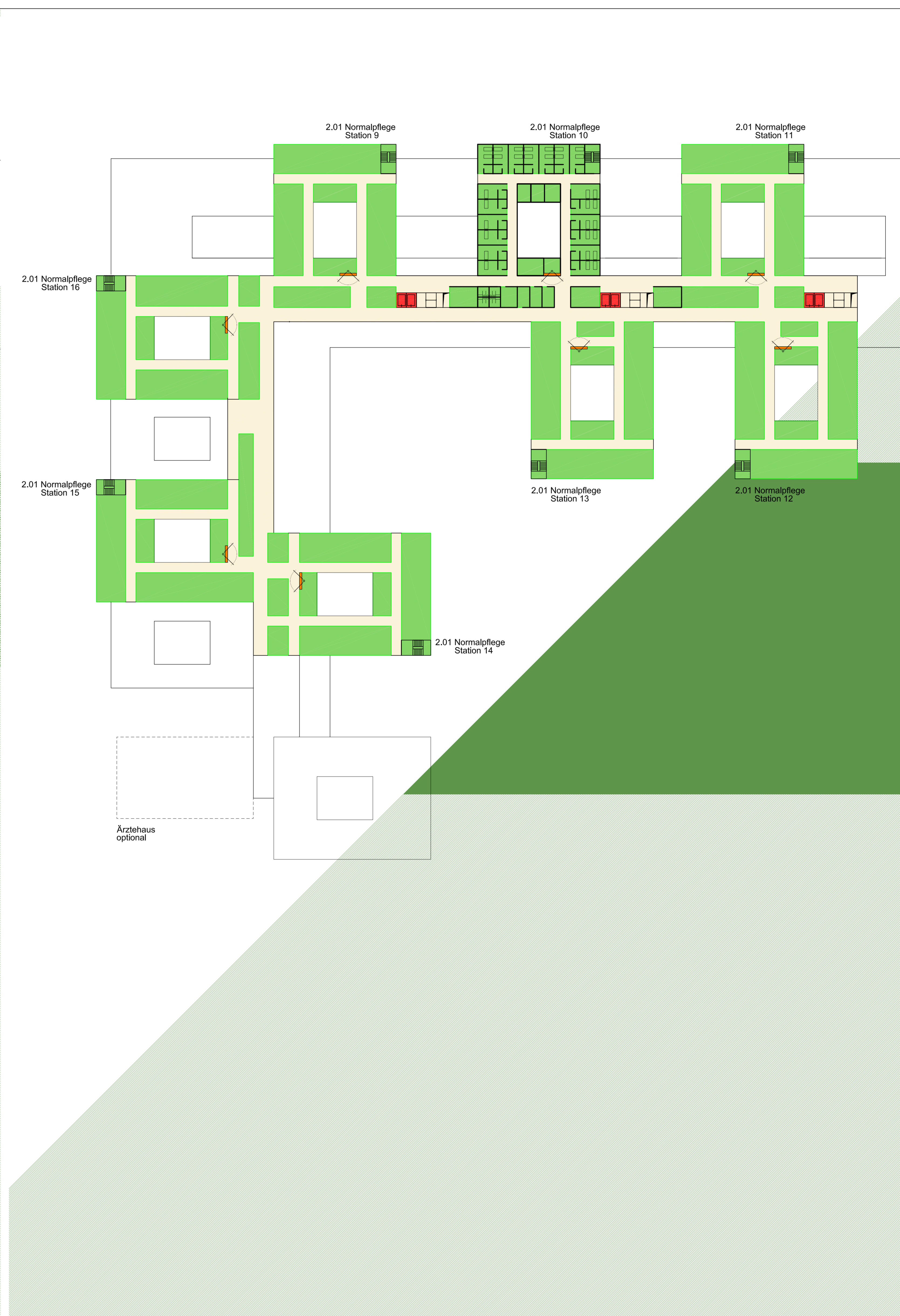
Grundriss 4.OG M1:500
