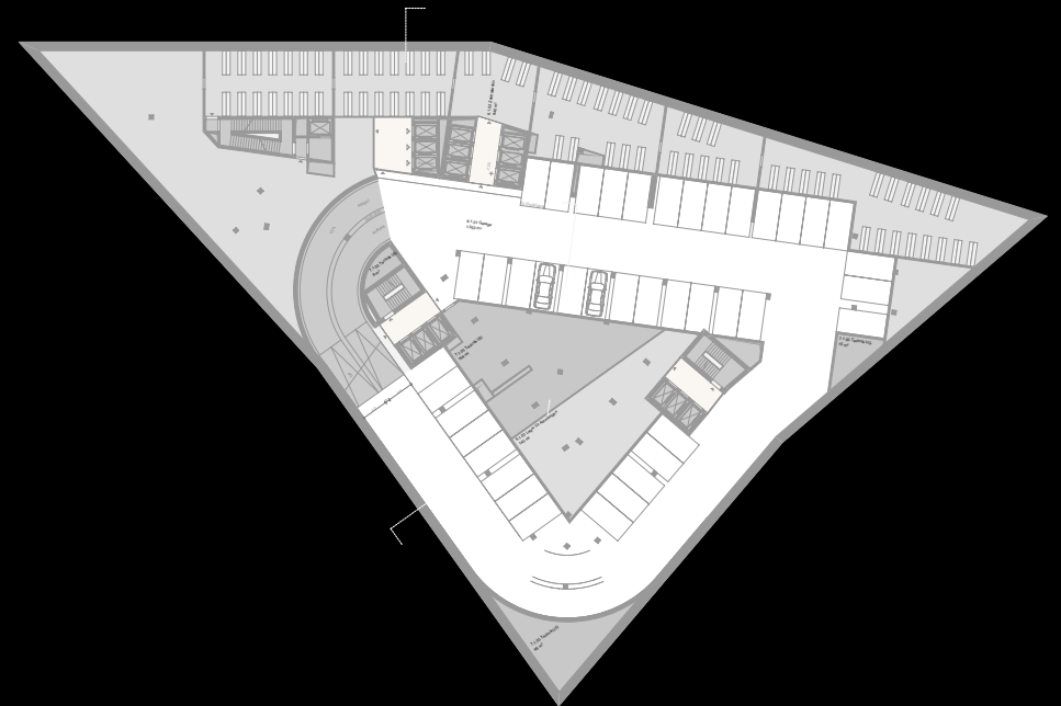
Grundriss 2.Untergeschoss M. 1.200
