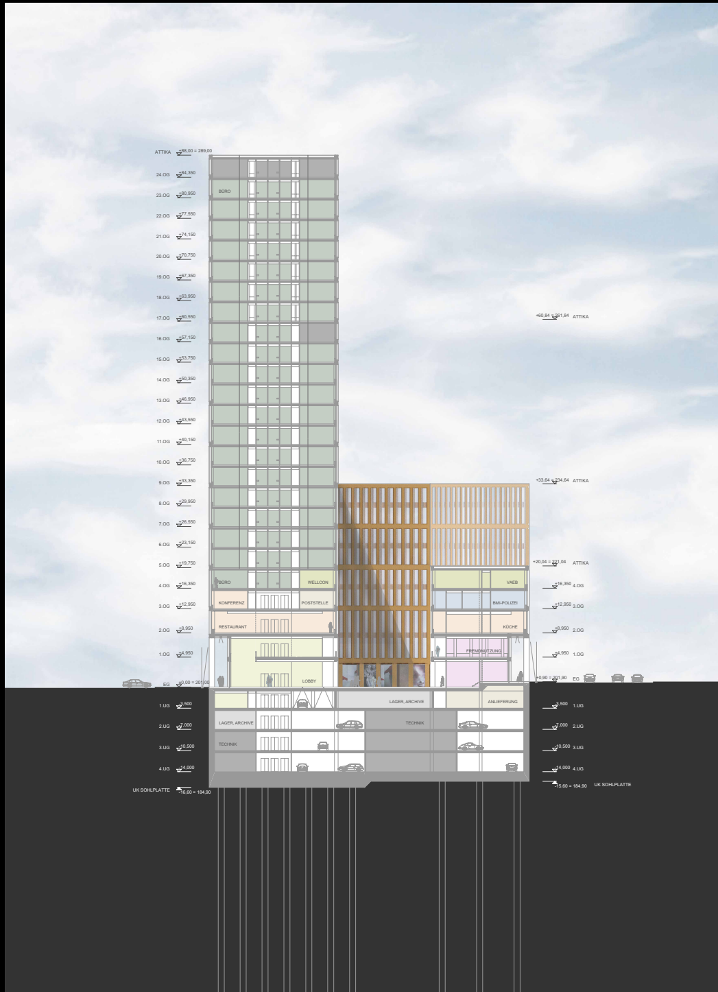
Schnitt M. 1.200
