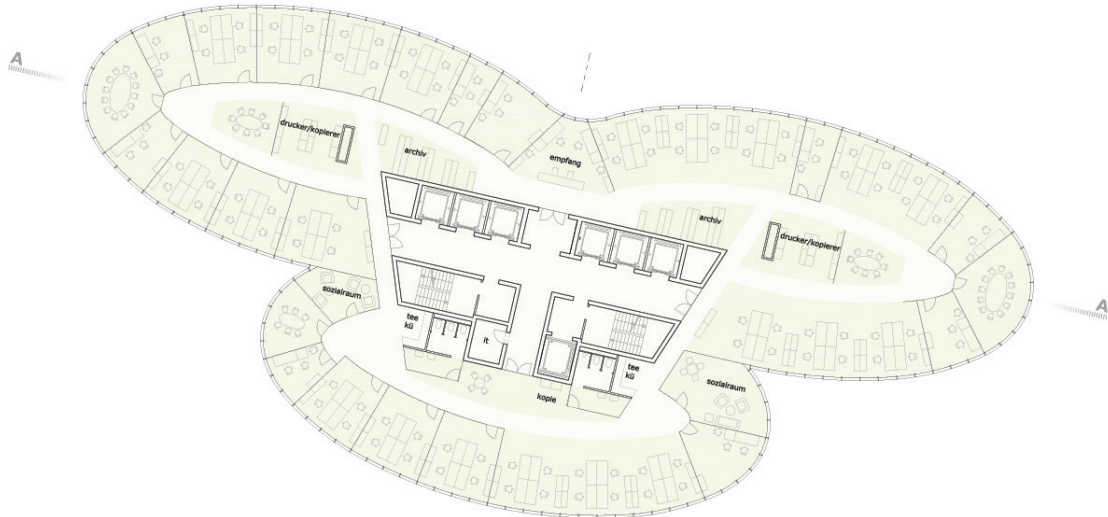
REGELGESCHOSS - VARIANTE B
