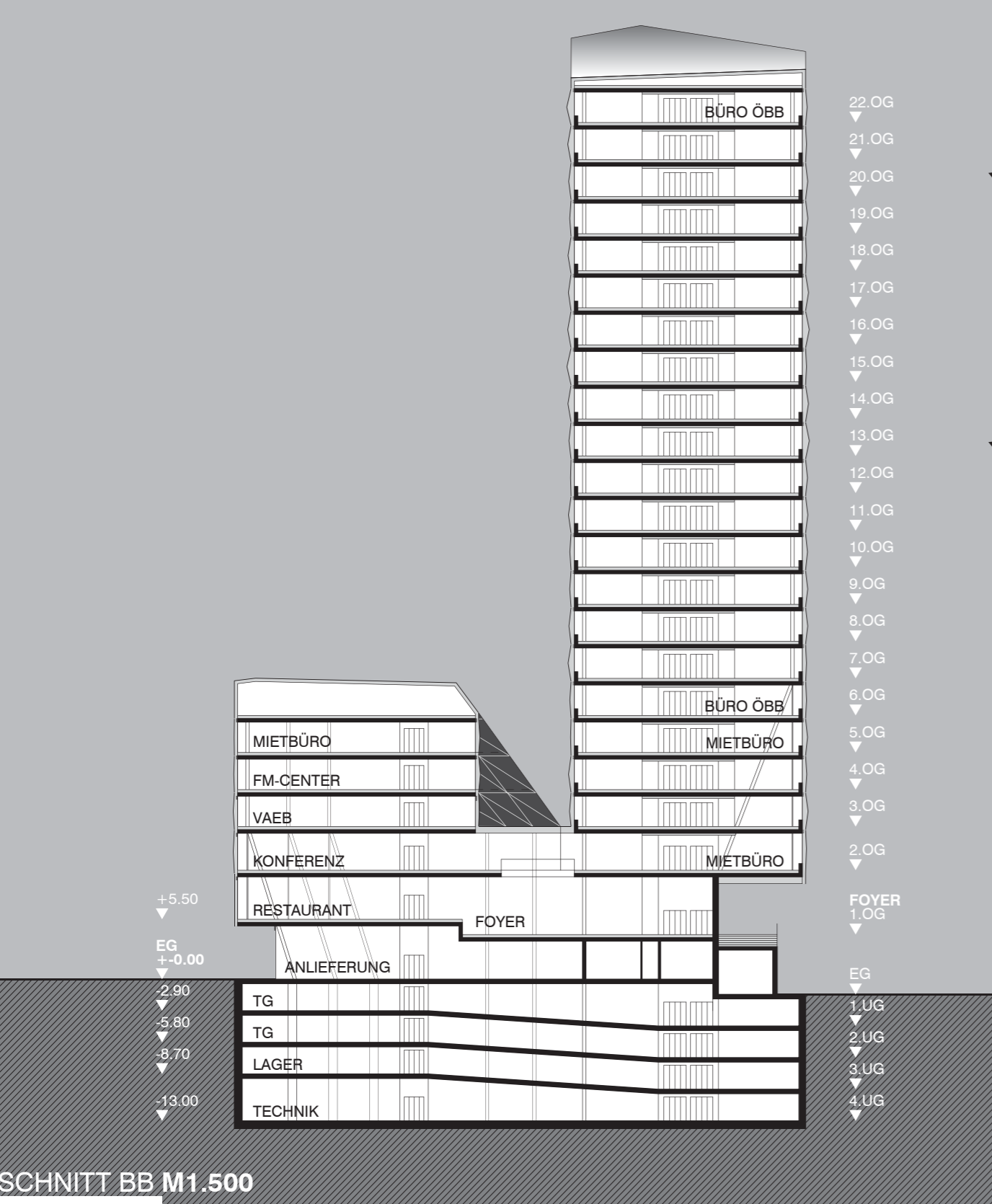
SCHNITT BB M1.500
