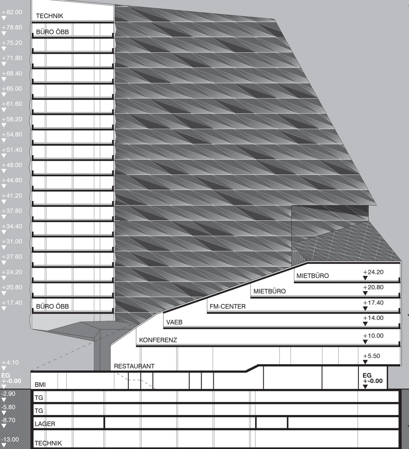
SCHNITT AA M1.500
