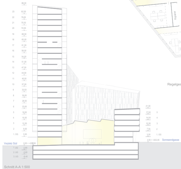
Schnitt A-A 1:500
