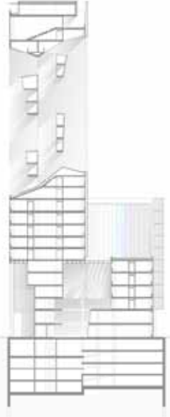
QUERSCHNITT 1:500
