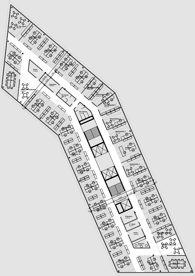
REGELGESCHOSS 9.-20.OG M 1:200 VARIANTE A
