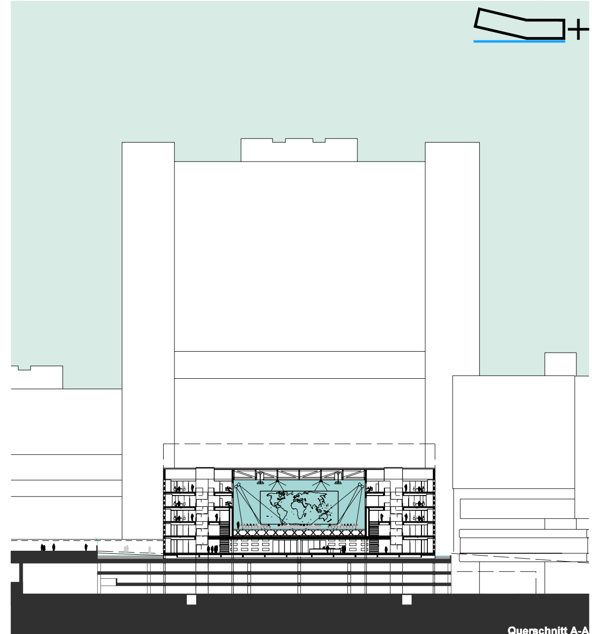
Querschnitt A-A
