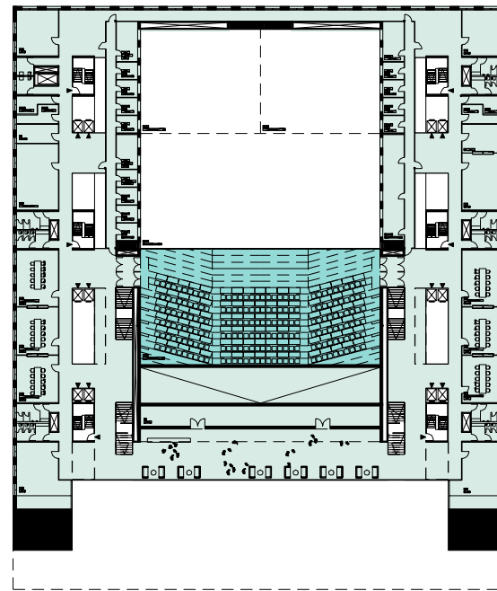
Ebene 02
