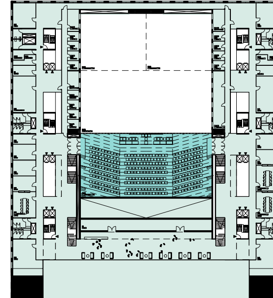
Ebene 02 - temporär
