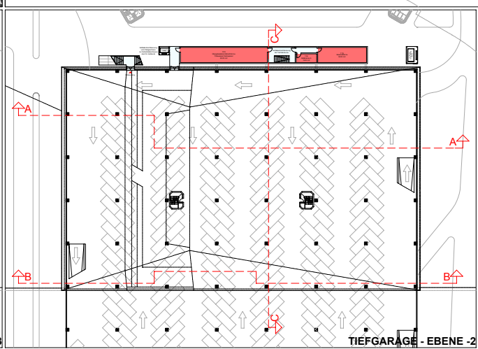
TIEFGARAGE - EBENE -2
