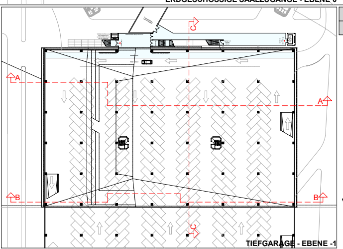
TIEFGARAGE - EBENE -1
