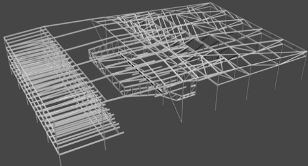
KONSTRUKTIONSSCHEMA
