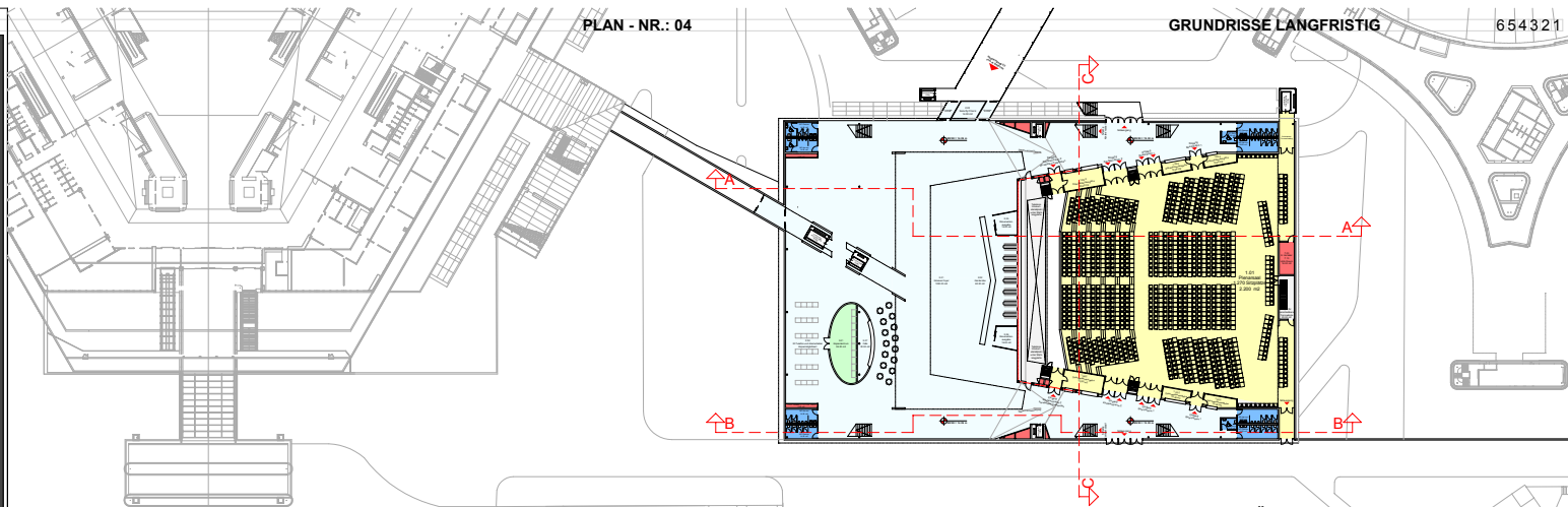
ERDGESCHOSSIGE SAALZÜGÄNGE - EBENE 0
