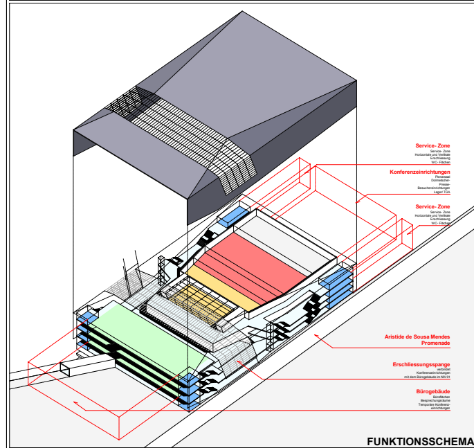
FUNKTIONSSCHEMA
