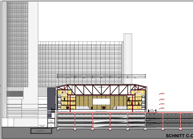
SCHNITT C-C
