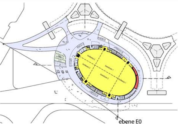
ebene E0
