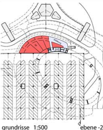
grundrisse 1:500
