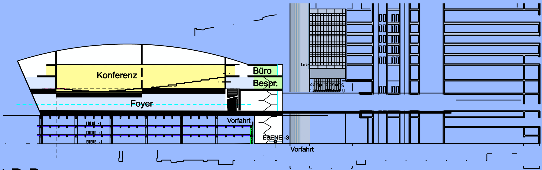
Schnitt B-B
