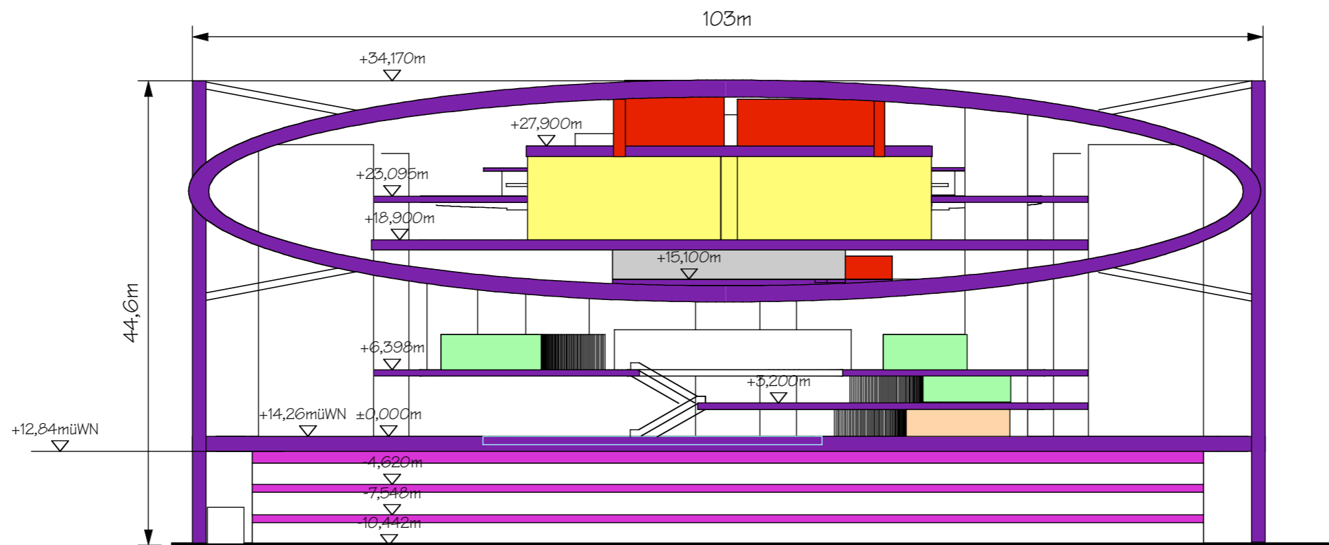
SCHNITTSCHNITT AA'
