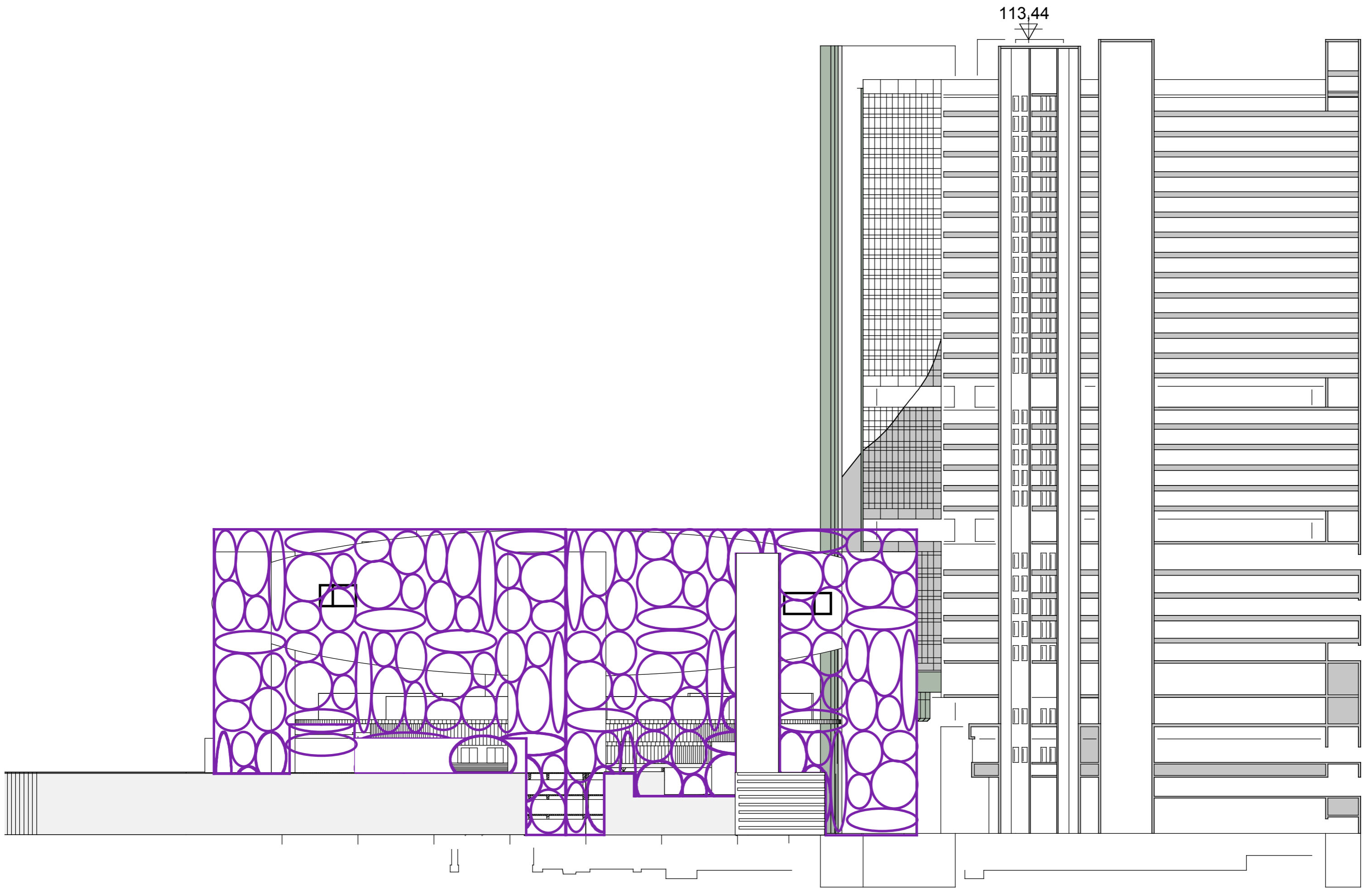
ANSICHT VON SW mit Fassade Kubus
